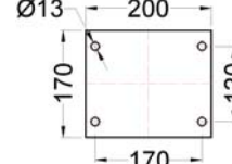
GDPAX / FDPAX larg. 4" GDPAXE / FDPAXE
